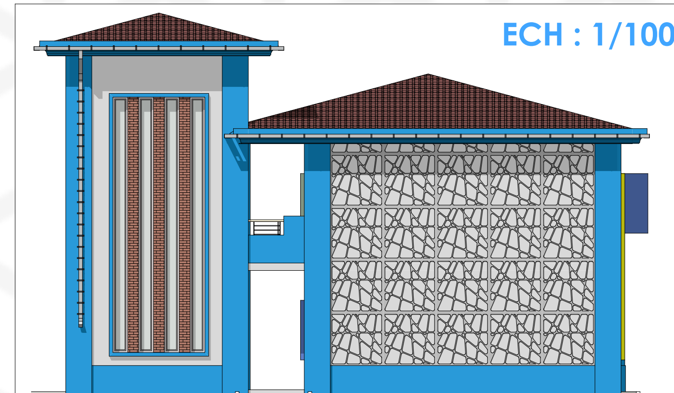
FACADE L.GAUCHE
